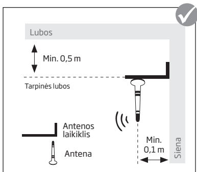
7 pav.: Tinkamas antenos montavimas prie lubų
