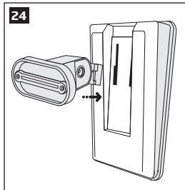
2.5. Įstatykite įrenginio laikiklį į įrenginio korpuso nugarinėje pusėje esančią angą
