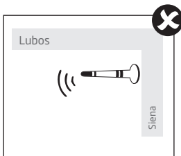
8 pav.: Neteisingas antenos montavimas prie lubų
