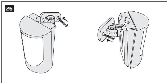
2.7. Pasirinkę tinkamą vietą įrenginio montavimui, medvaržčiais pritvirtinkite laikiklį prie sienos
